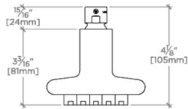
SIDE VIEW SCALE: 3"=1'-0"
