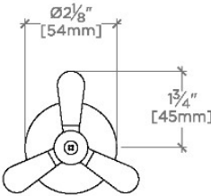
FRONT VIEW SCALE: 3"=1'-0"
