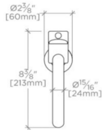
TOP VIEW SCALE: 1 1/2" = 1'-0"
