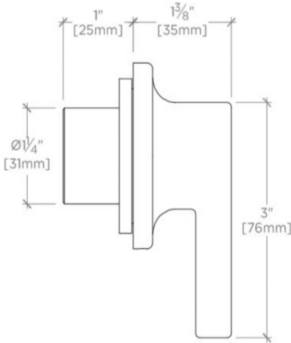
SIDE VIEW SCALE: 6"=1'-0"
