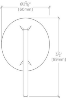
FRONT VIEW SCALE: 6"=1'-0"
