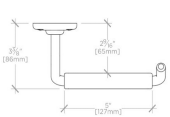
TOP VIEW SCALE: 3"=1'-0"
