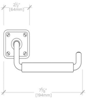
FRONT VIEW SCALE: 3"=1'-0"
