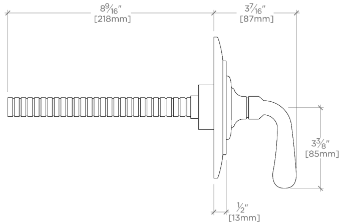
SIDE VIEW SCALE: 3"=1'-0"
