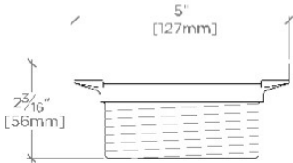
FRONT VIEW SCALE: 3"=1'-0"
