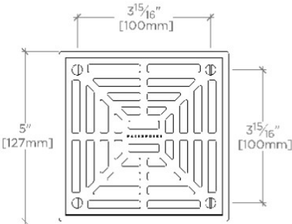
TOP VIEW SCALE: 3"=1'-0"
